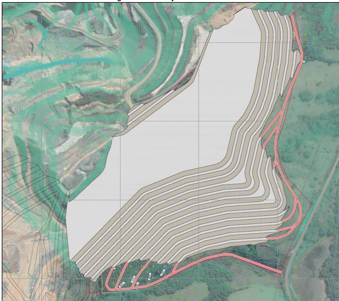
Figura 5.4 – Arranjo Geral – PDE 08
