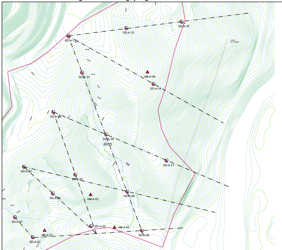
Figura 5.3 - Investigação geotécnica - Planta
