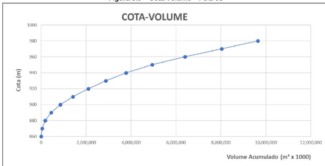
Figura 5.5 – Cota Volume – PDE 08
