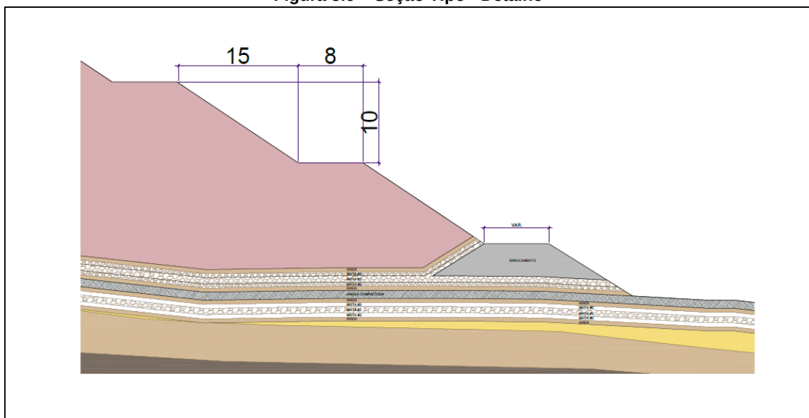
Figura 5.6 – Seção Tipo - Detalhe
