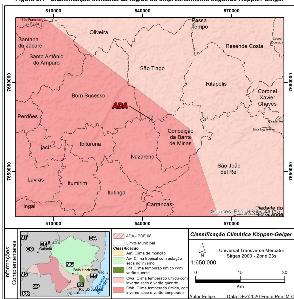
Figura 3.4 - Classificação climática da região do empreendimento segundo Köppen-Geiger
