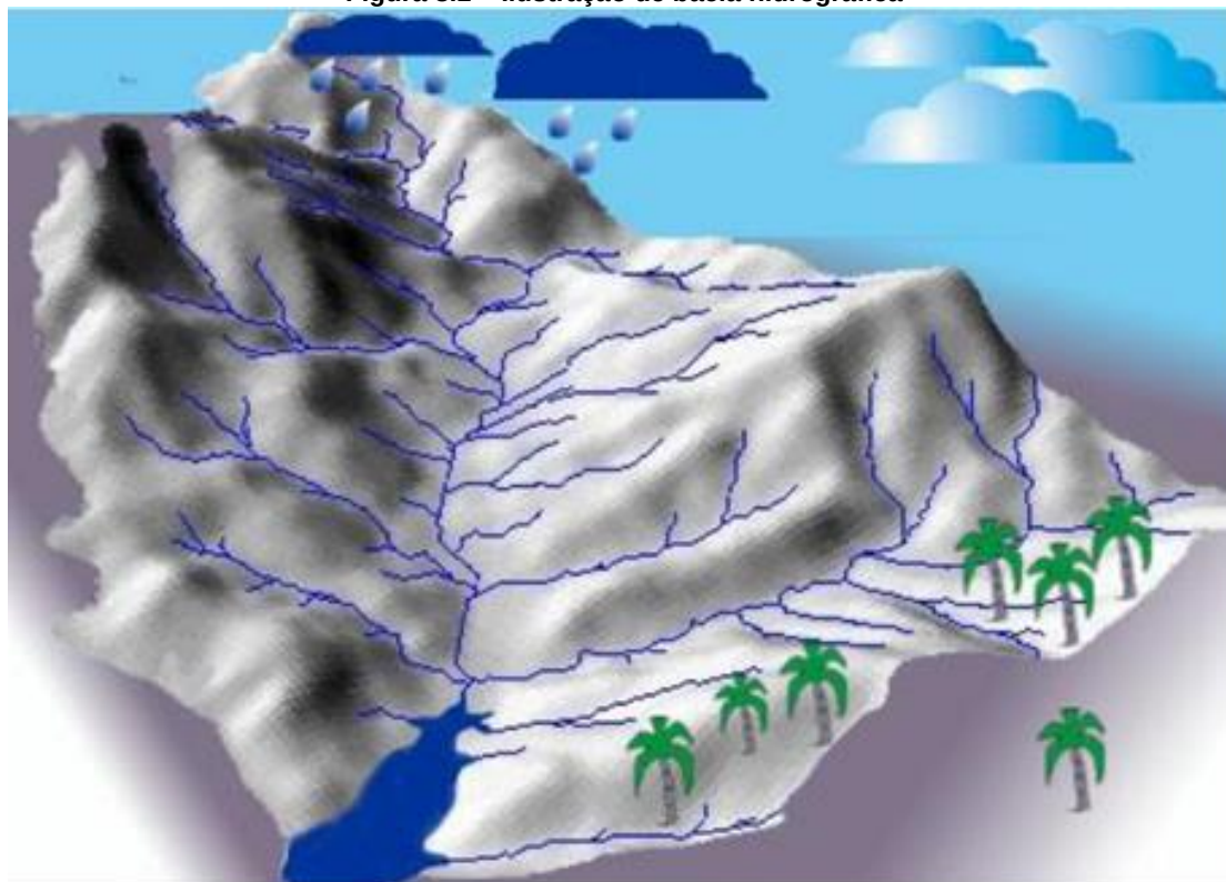
Figura 8.1 – Ilustração de bacia hidrográfica
